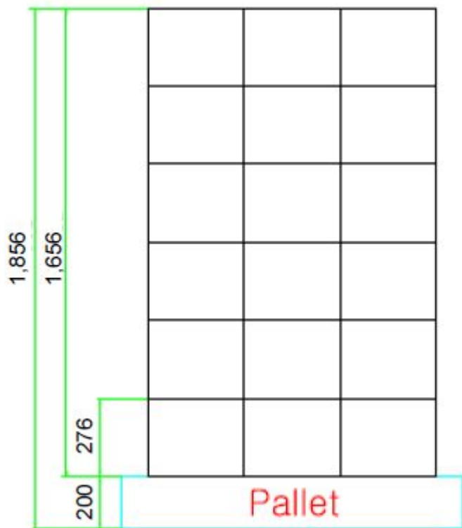
正面図
