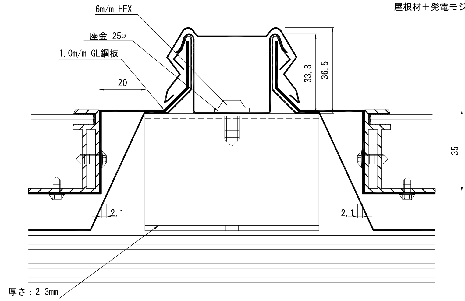
1:1 A部分拡大図
