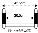
HKM-110 (固定型・ミニタイプ前輪固定キャスター付)
