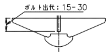
断面詳細図
