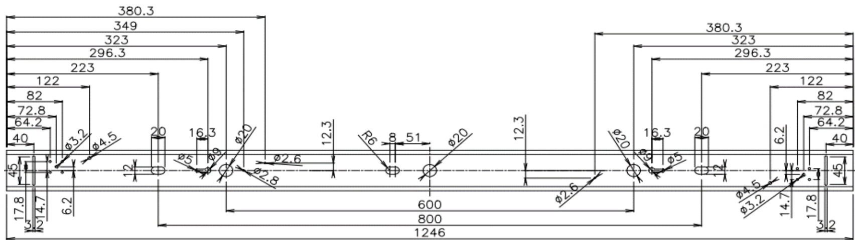
取付図
