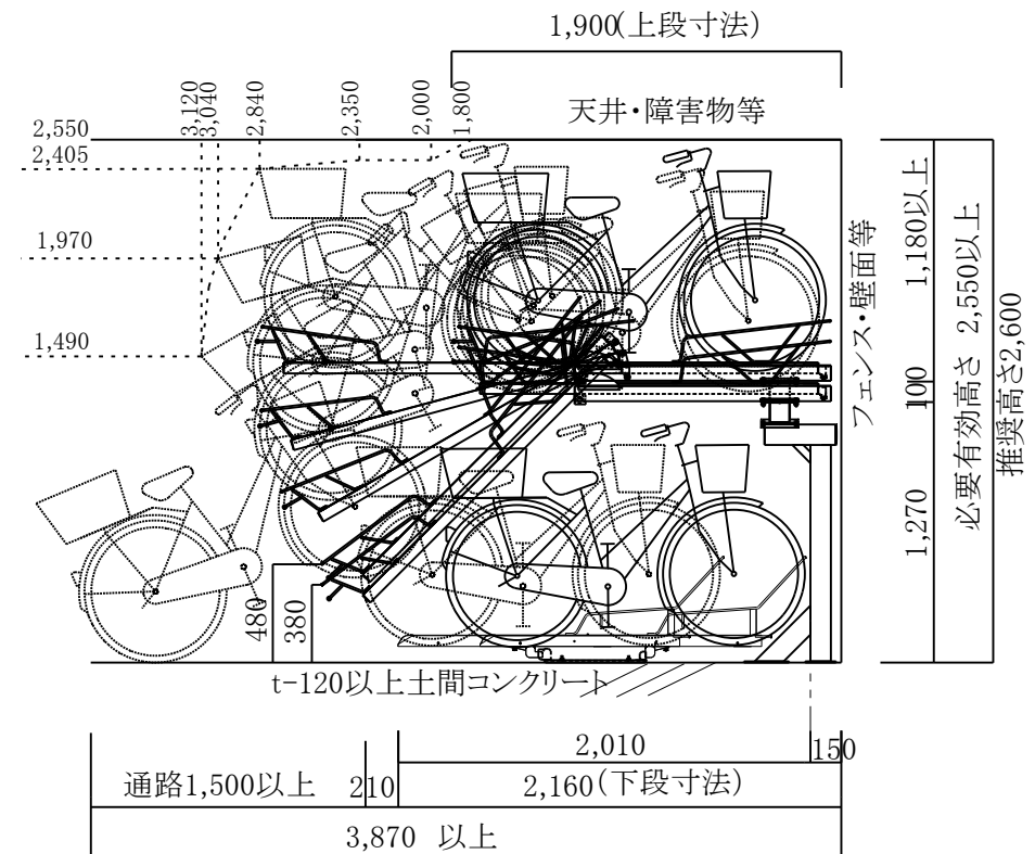
上段ラックMCY-GU型 (450P)/下段スライドラックMCY-S2型 (300P) 側面図
