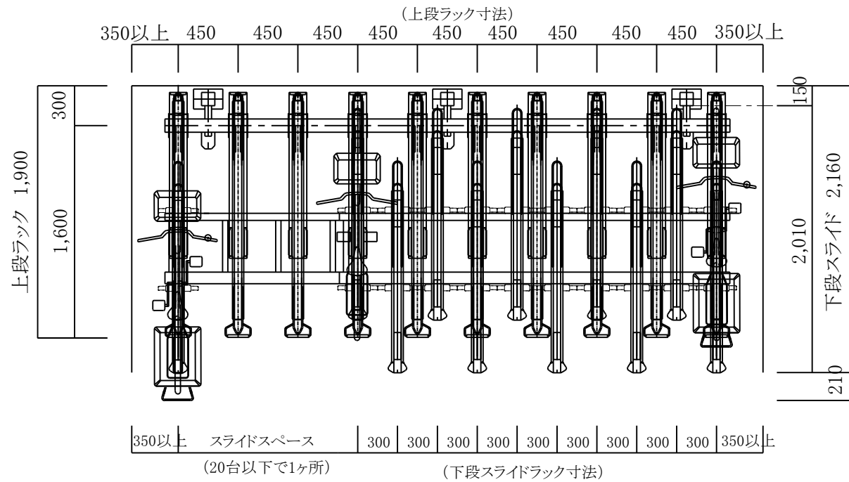
上段ラックMCY-GU型 (450P)/下段スライドラックMCY-S2型 (300P) 平面図
