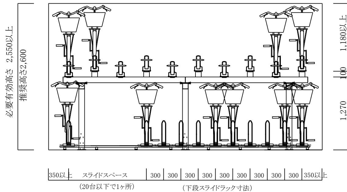
上段ラックMCY-GU型 (450P)/下段スライドラックMCY-S2型 (300P) 正面図
