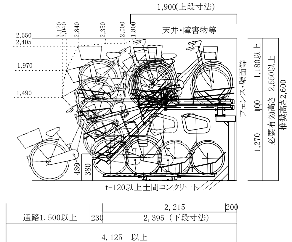
上段ラックMCY-GU型 (450P)/下段スライドラックMCY-S4型 (300P) 側面図
