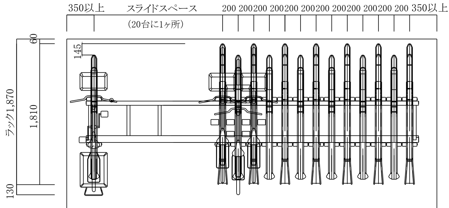
省スペーススライド式ラック MCY-S3型 (200P) 平面図
