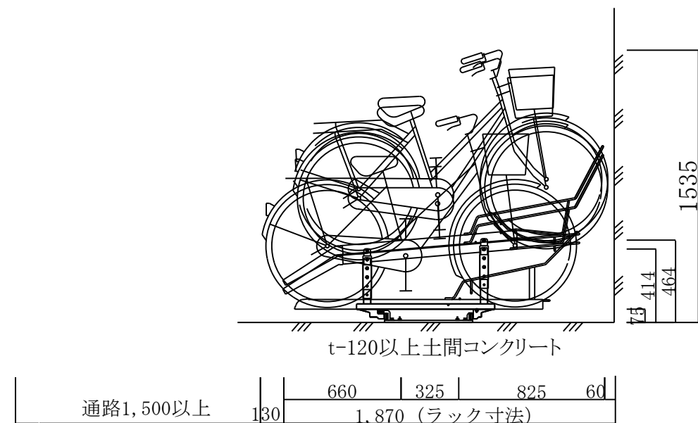
省スペーススライド式ラック MCY-S3型 (200P) 側面図
