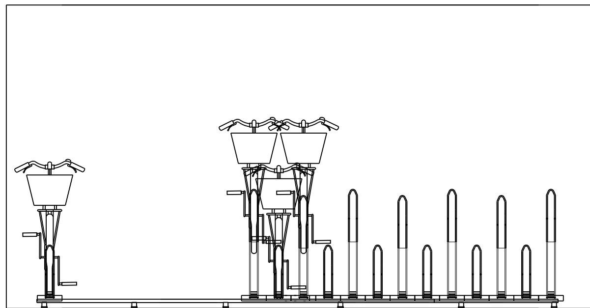
スライド式サイクルラック MCY-S3型 (200P) 正面図
