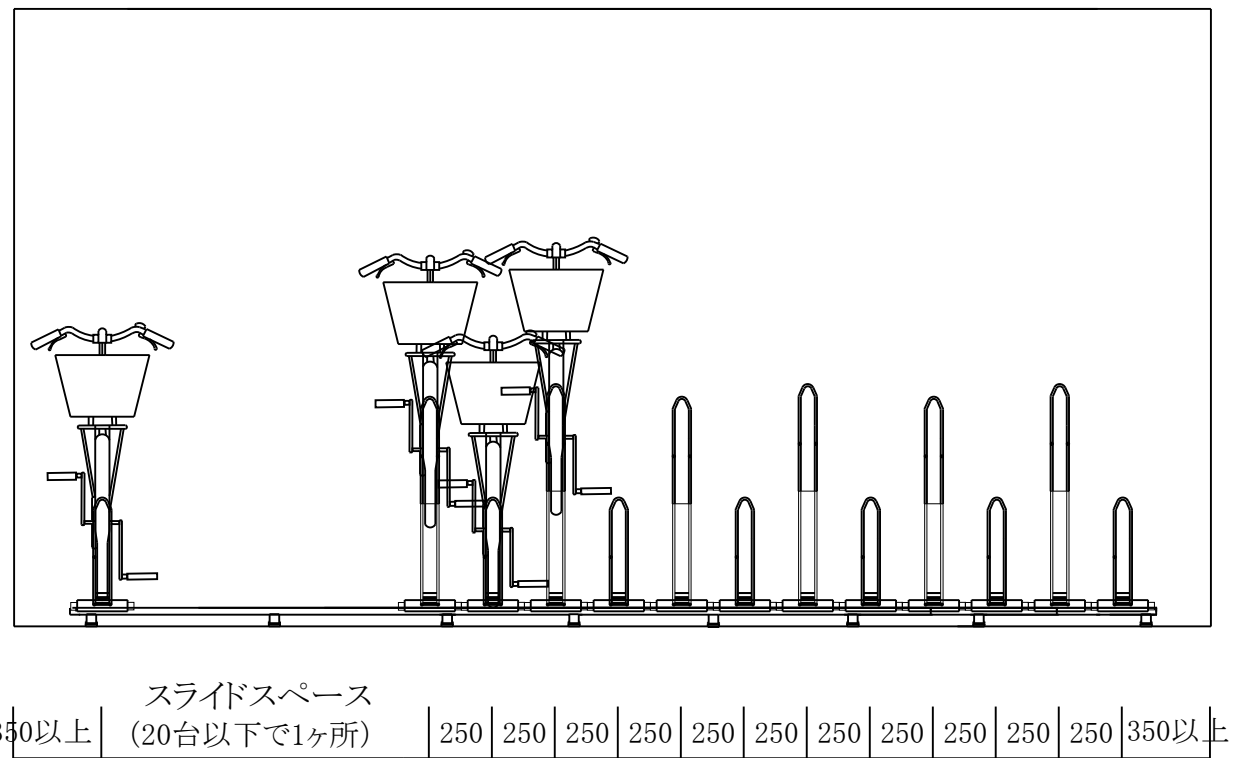
スライド式サイクルラック MCY-S3型 (250P) 正面図
