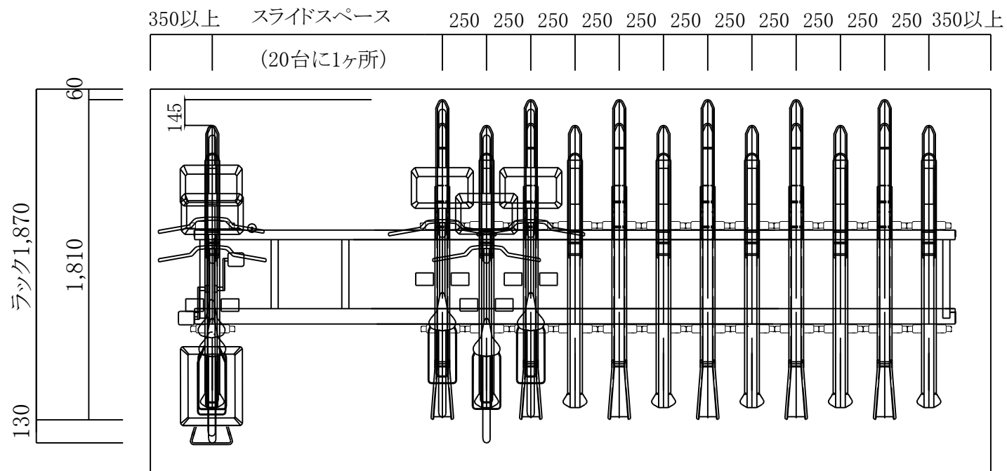
省スペーススライド式ラック MCY-S3型 (250P) 平面図
