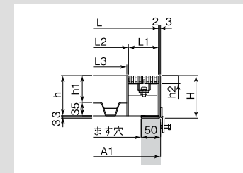
盗難・騒音防止フック部 断面図
